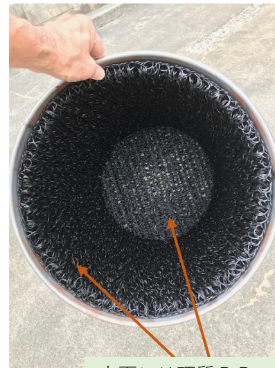
内面には硬質PP 無数のR形状でフィルター保護 フィルターの通水の為の空気層を形成
